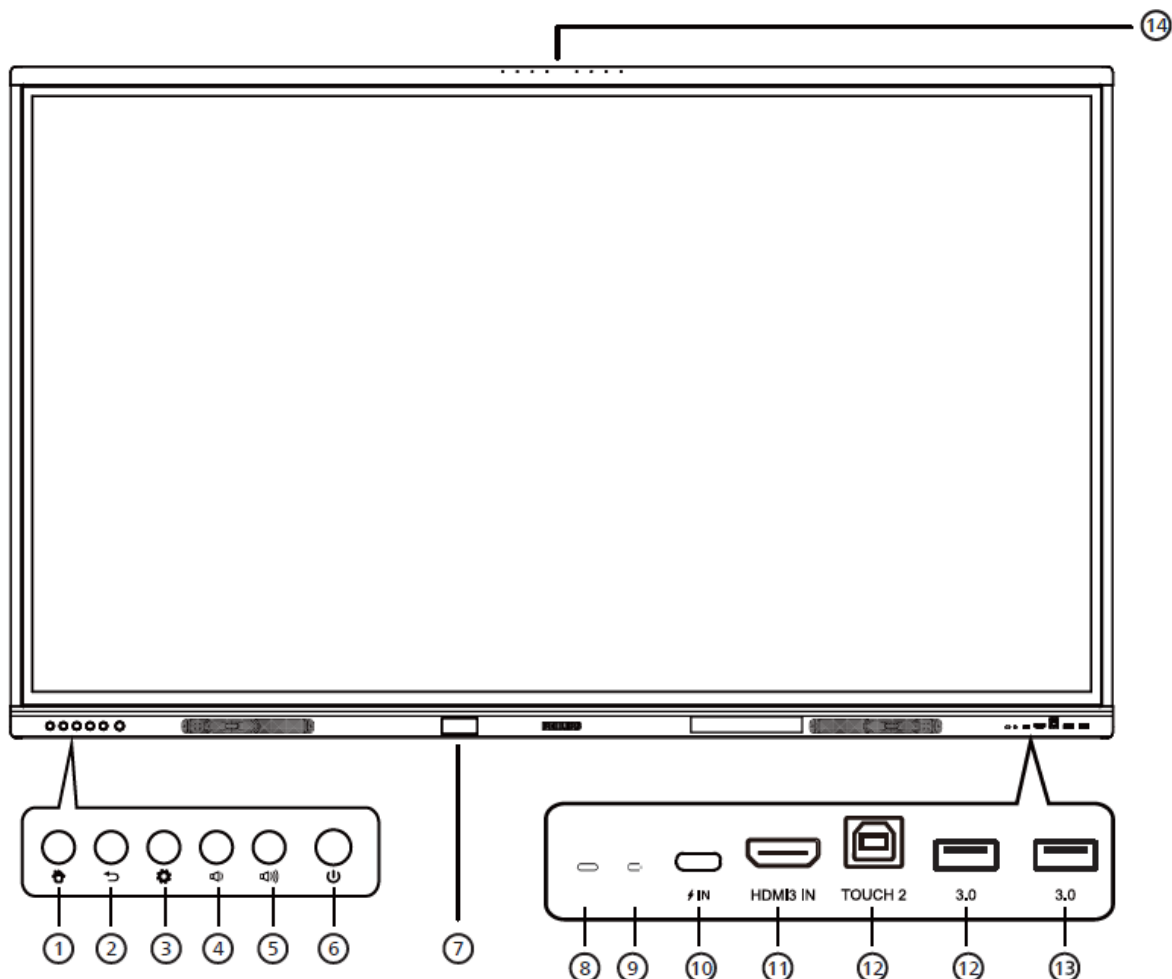
Slika 1. Prednja strana zaslona
