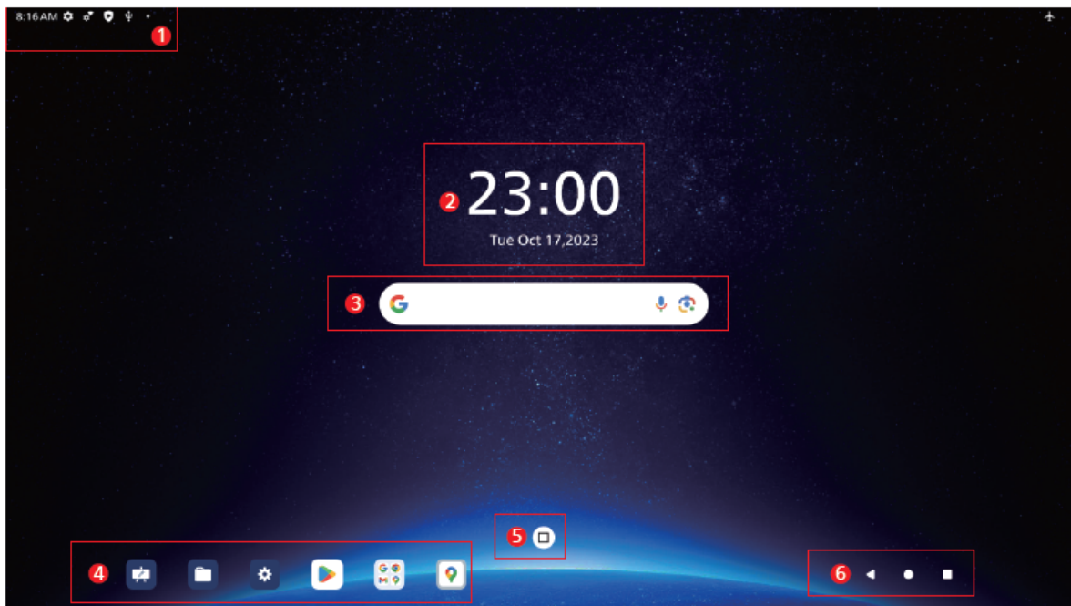
Slika 4. Početni zaslon
