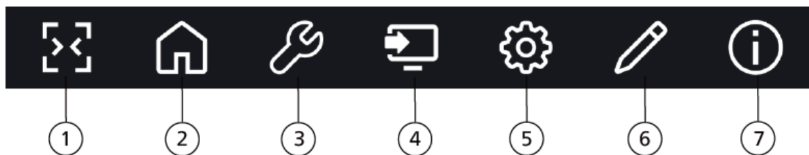
Slika 4. Plutajuća traka
