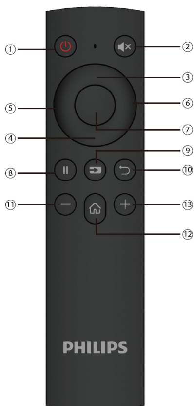
Slika 3. Daljinski upravljač
