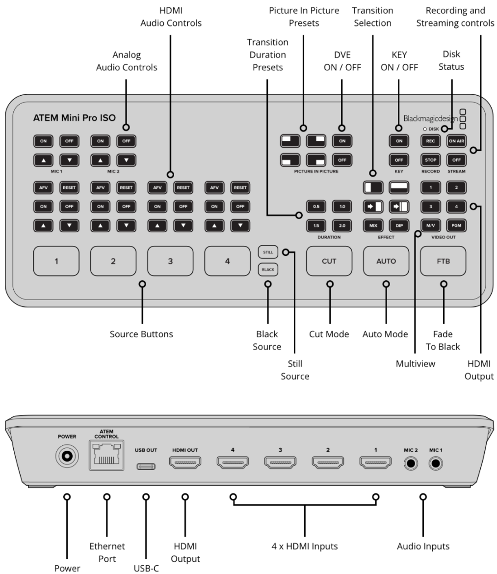
Slika 1. Pregled ATEM Mini PRO ISO
