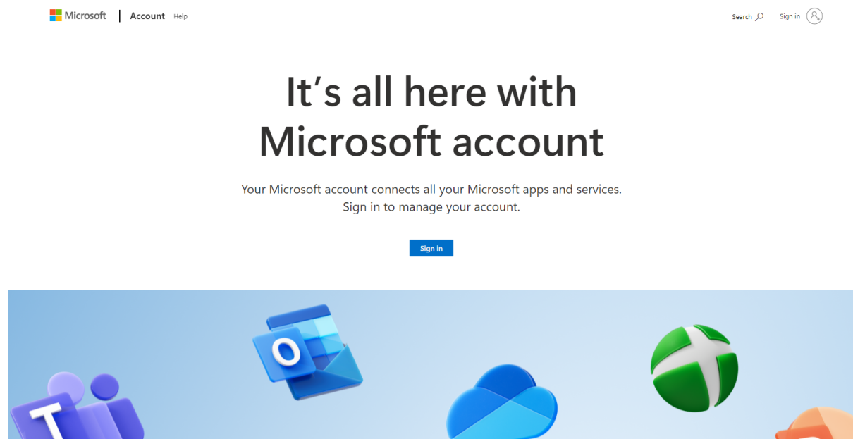
Slika 4. Microsoft račun
